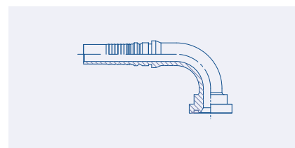
Interlock 90° Swept SUPERCAT Flange
