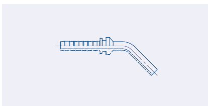
45° Swept Metric Standpipe (BEL 45)
