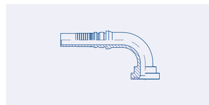
Interlock 90° Swept SAE 6000 PSI (code 62) Flange (SFS 90°)
