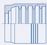
NON SKIVE Balfit® 4 Spiral Ferrule 20.NS4
