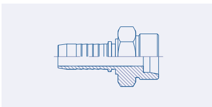
Male Metric French Serie 24° Cone Seat (AGF)
