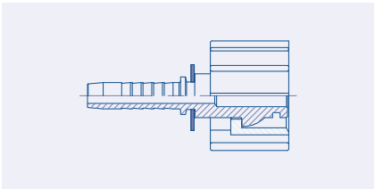
Balwash Female Swivel (Karcher) 23.6213
