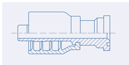
Straight SuperCAT Flange - CS
