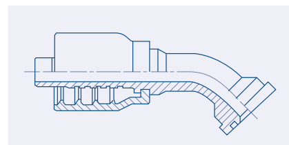
45° Elbow SAE 6000 PSI Code 62 Flange - PH45
