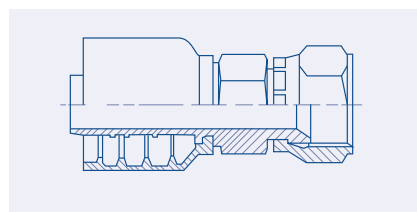
JIS 30° Female Swivel - JIS
