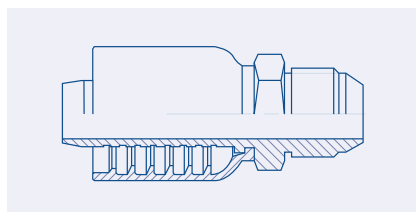
Male SAE 45° Rigid - MX
