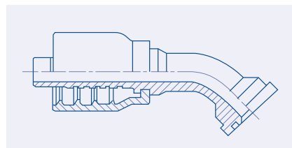
45° Elbow SuperCAT Flange - CS
