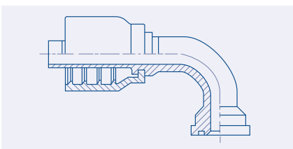
90° Elbow SuperCAT Flange - CS
